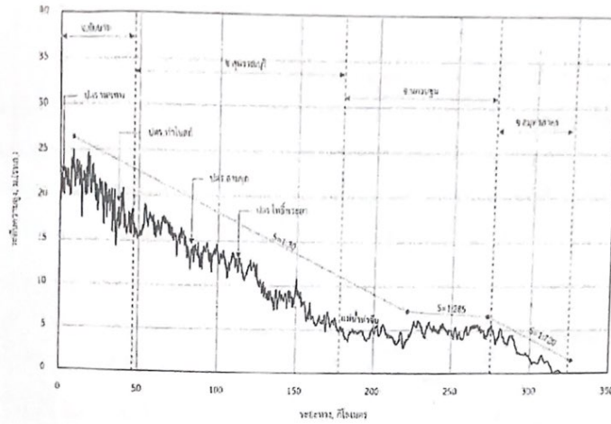
รูปที่ 2.1.1-2 รูปตัดตามยาวแม่น้ำท่าจีนแสดงความลาดชันผืนน้ำ
